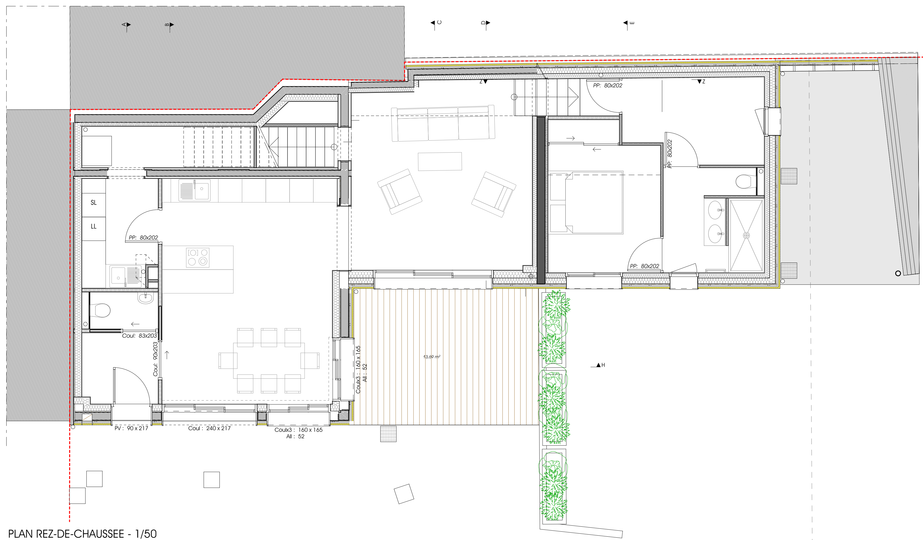
PLAN REZ-DE-CHAUSSEE - 1/50
